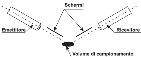
Fig. 1 Schema di funzionamento del sensore
